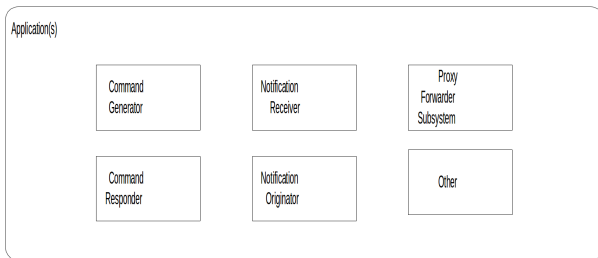
Figur: SNMPv3 applikationer[3]
