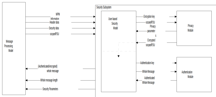
Figur: Utgående meddelanden [3]
