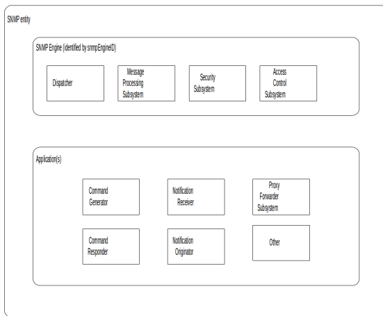
Figur: SNMPv3 arkitektur överblick [3]
