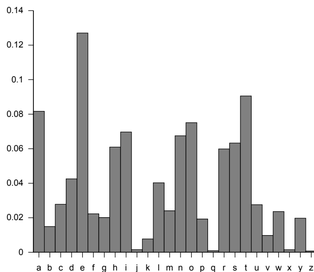
Figur 2: En överblickande graf över sannolikhetsfördelningen för den stokastiska variabeln E . Bild: [WPa].
